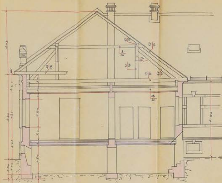
B. METSZET 1:50
