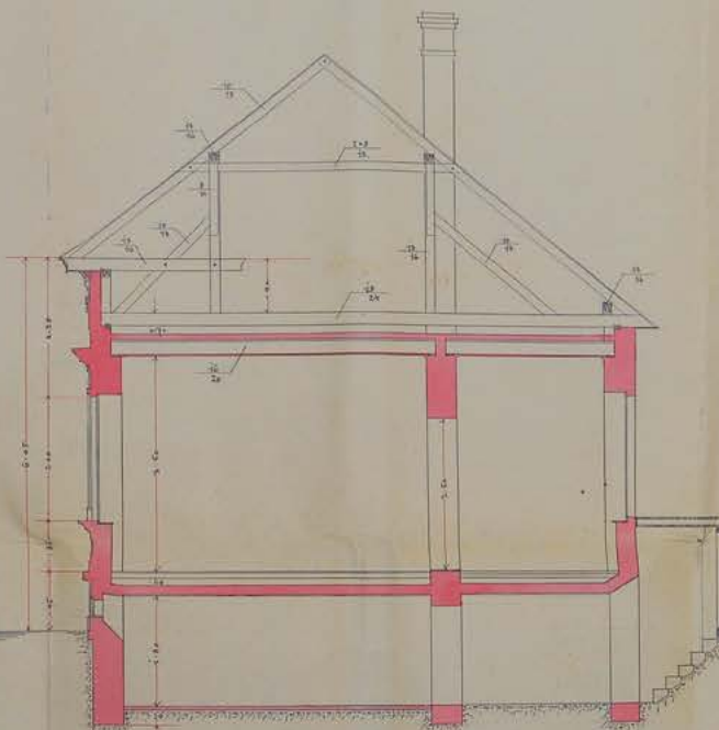
a-b fűtőcsatlakozás 1:50.
