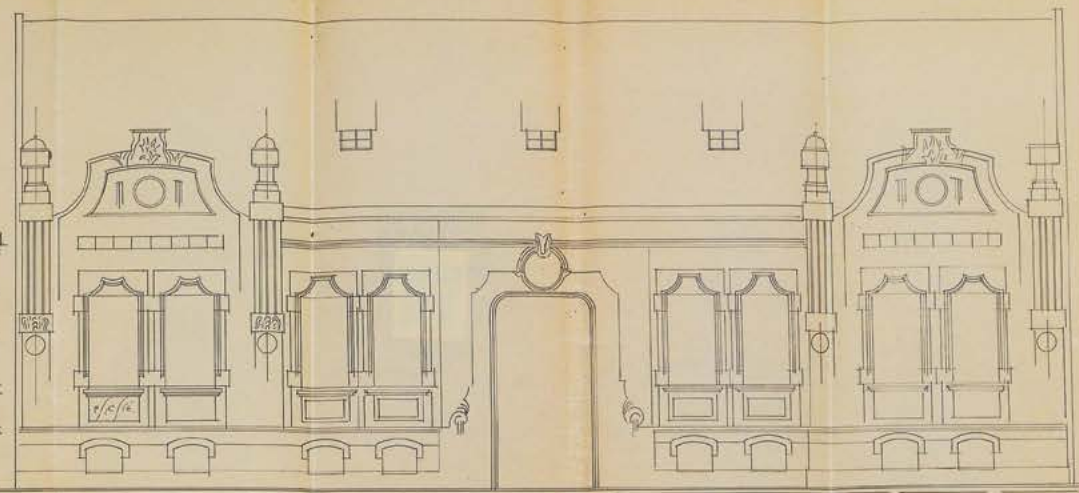
HOMLOKZAT 1:50
