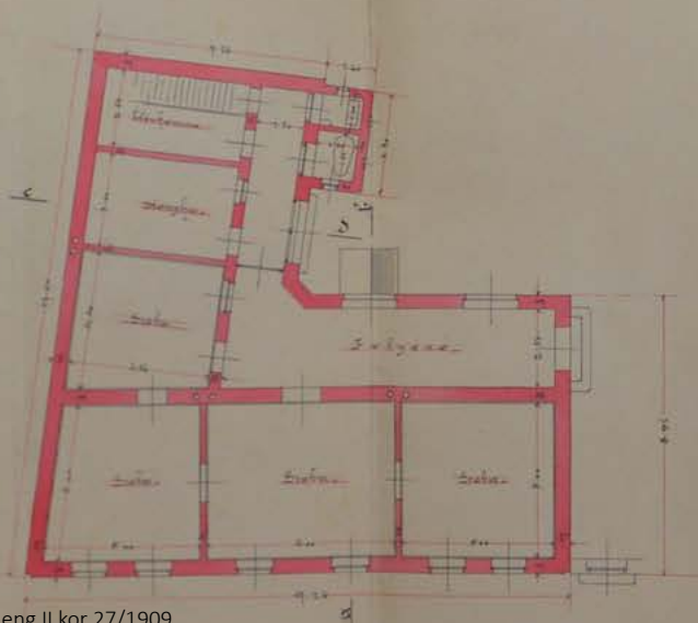
Földszinti alaprajz 1:100.
